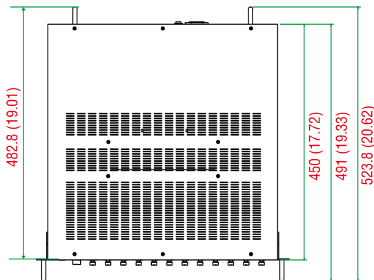
上面図
